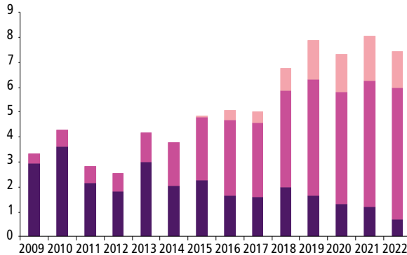
رسم بياني 6.2.1: إنتاج الكهرباء من مصدر متجدد (بآلاف جيغاواط الساعة)
